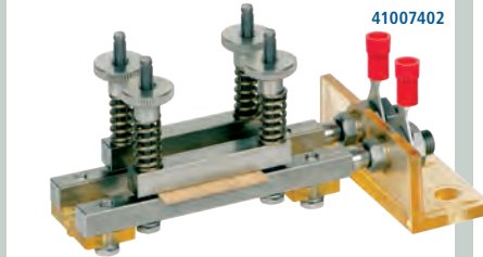
ANSICHT Anschlusswinkel [links] mit eingestecktem UGL-Elektrodenhalter und UGL-Sensor [rechts]
