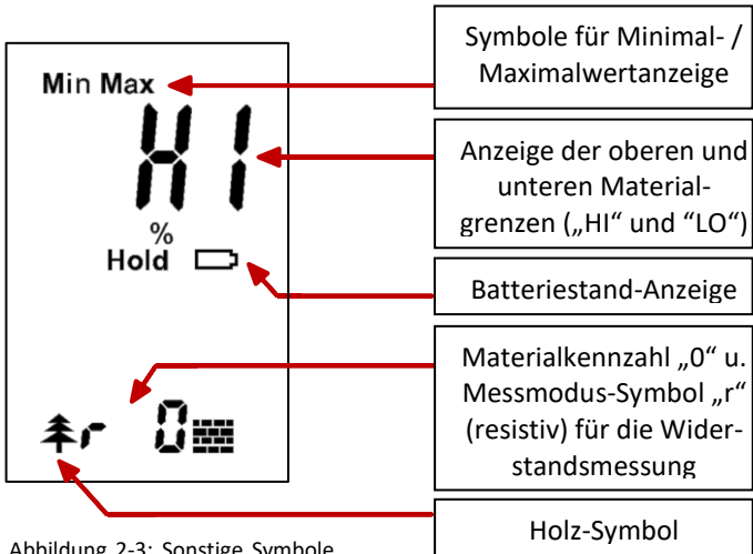
Abbildung 2-3: Sonstige Symbole resistive Messung
