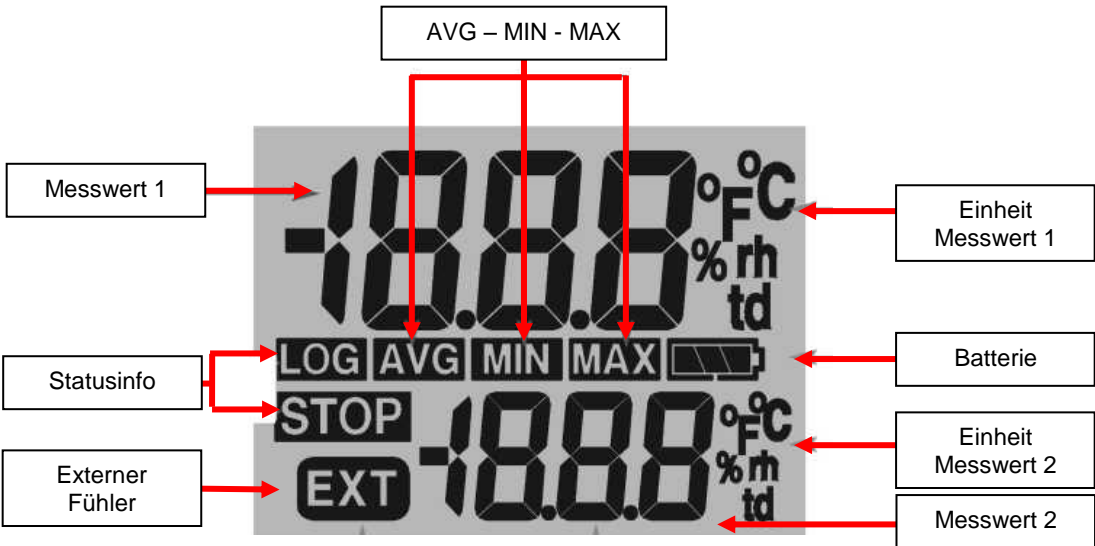
Abbildung 1-4 Displaysymbole Klima 30
