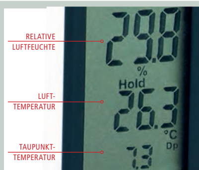
DETAILANSICHT DISPLAY
